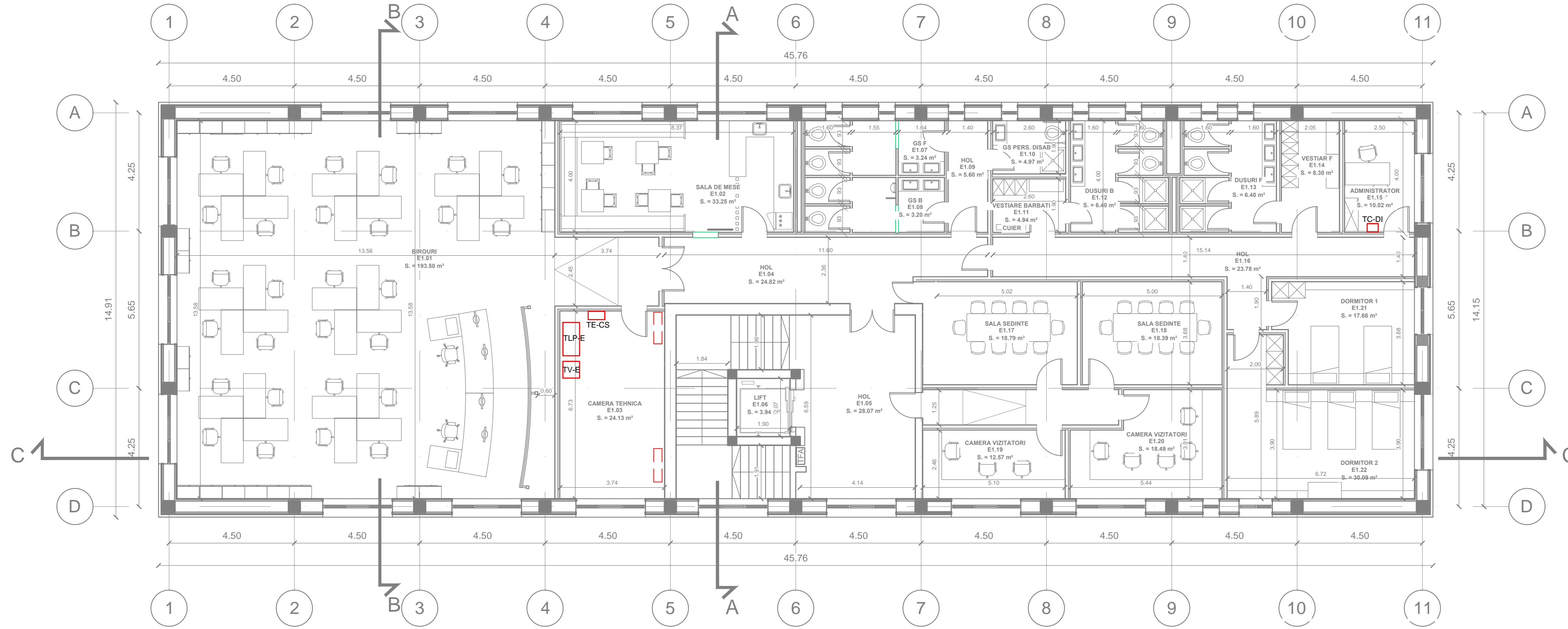
PLAN ETAJ 1
