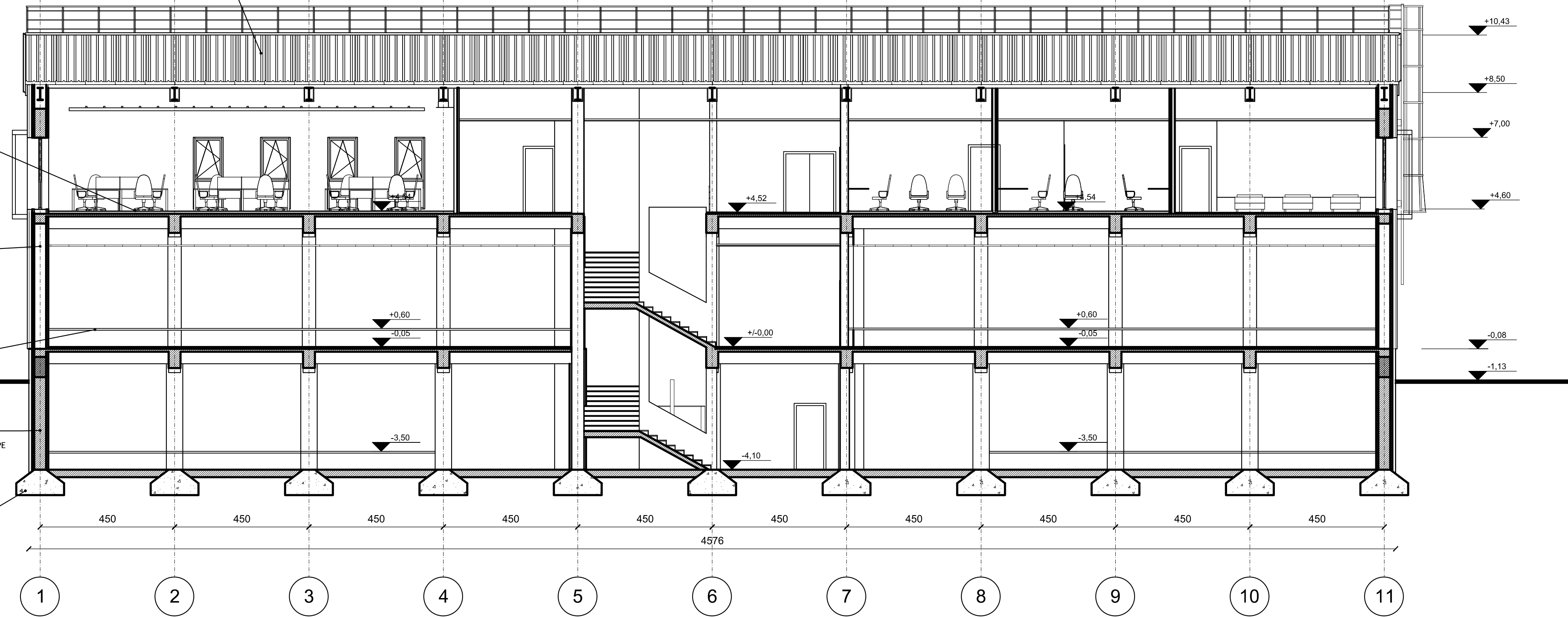
SECȚIUNE LONGITUDINALĂ C-C
